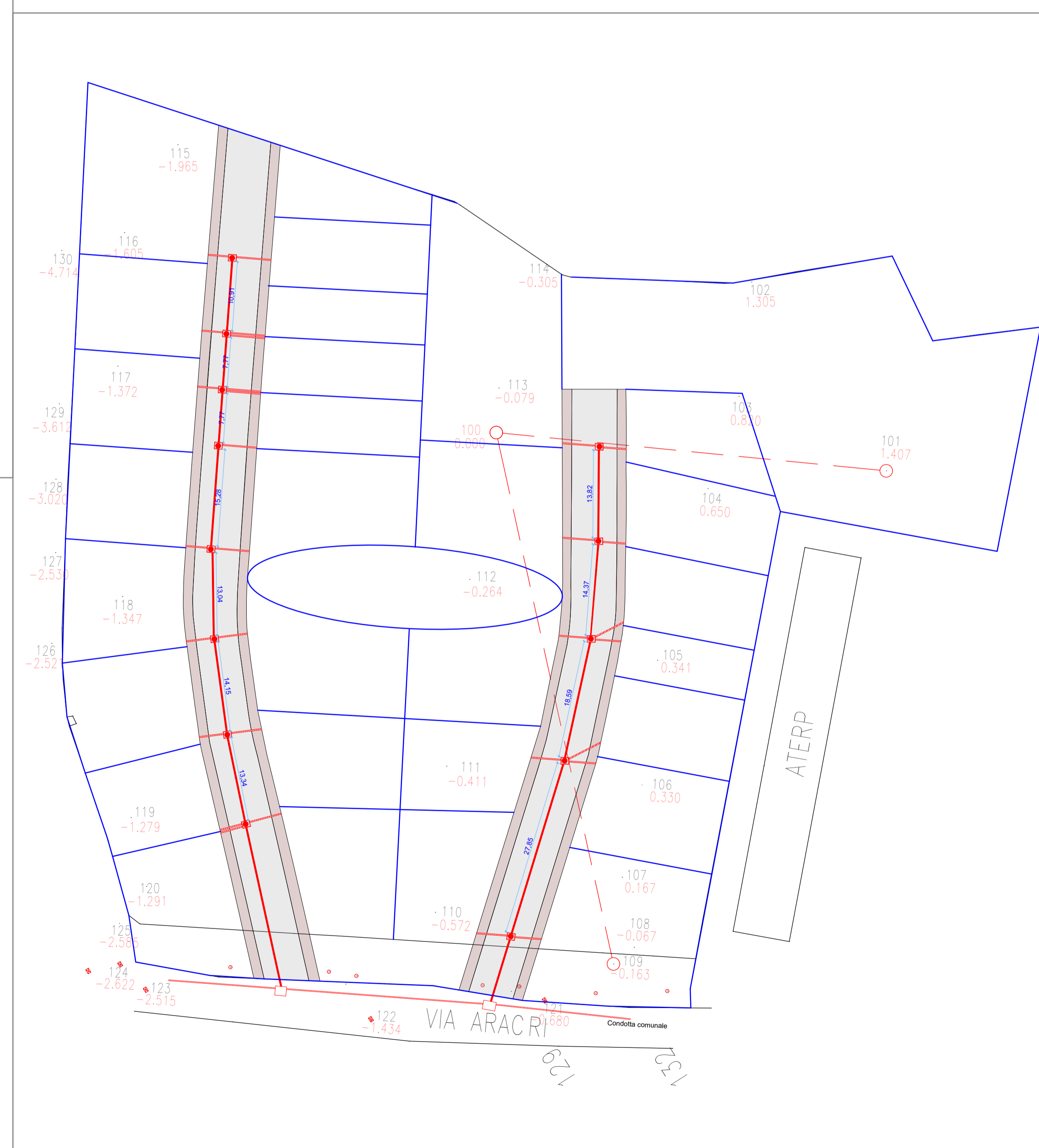
Planimetria condotta acque nere sc 1:500
